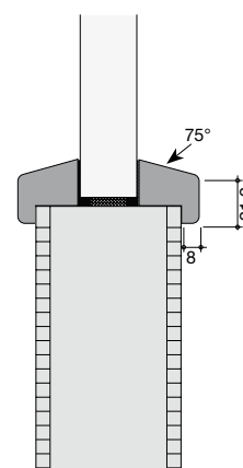
Schnittzeichnung Glasleiste Quadra
