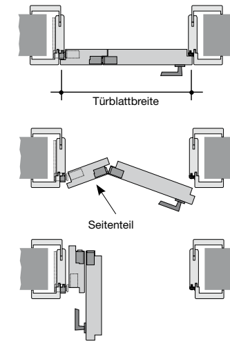
Schnittzeichnungen | Falt-Türelement
