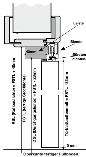
Maßangaben | Falt-Türelement
