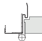
■ VARIANTE: stumpf (VX-Bandaufnahme erforderlich)
