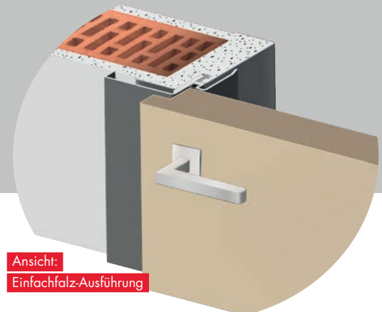
■ Stahl-Eckzarge SEZ auf Stahlzarge
