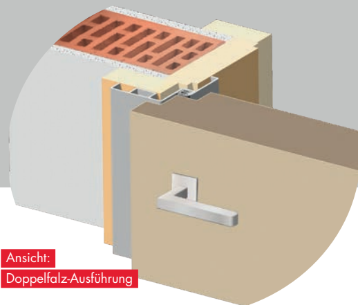
■ Stahl-Sanierungszarge SSEZ auf Holzstock
