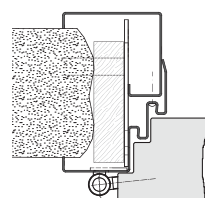
■ Montage: Mauerwerk
