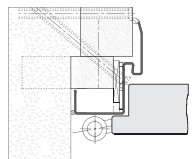
■ Montage: Holzstock Wandnische mit aufliegendem Spiegel
