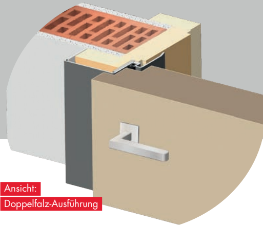
■ Stahl-Eckzarge SEZ auf Holzstock
