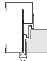
■ VARIANTE: stumpf (VX-Bandaufnahme erforderlich)
