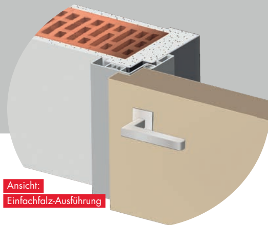
■ Stahl-Sanierungszarge SSEZ auf Stahlzarge
