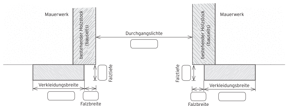
Maßaufnahme-Skizze 2)
