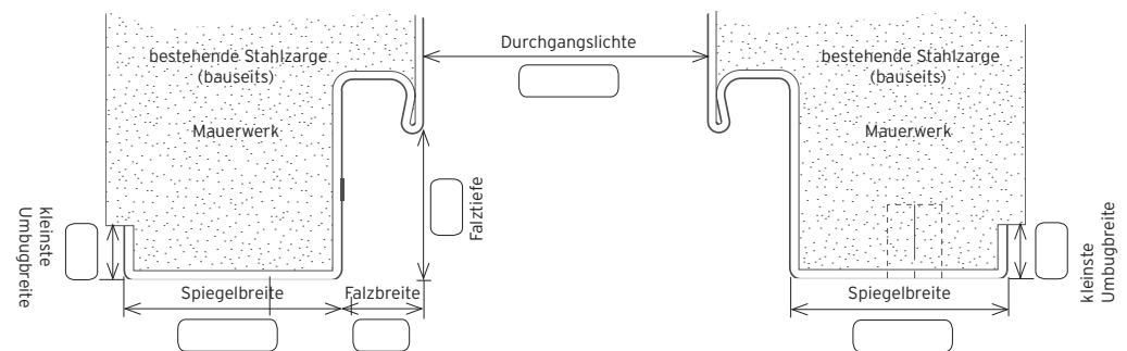
Maßaufnahme-Skizze 2)
