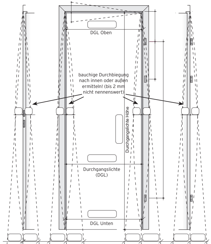
Maßaufnahme-Skizze 1)
