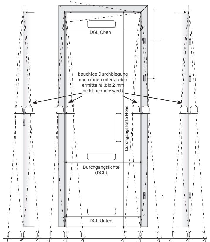
Maßaufnahme-Skizze 1)
