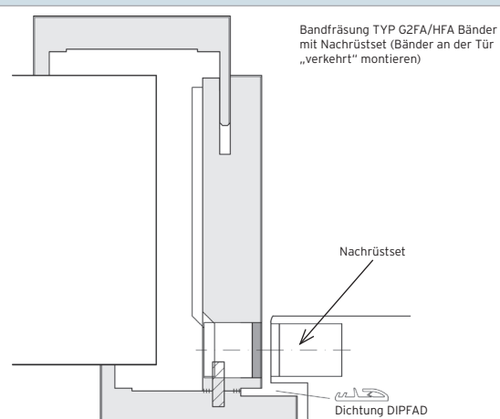
Bild 20 (Querschnitt Nachrüstset/Distanzhalter)
